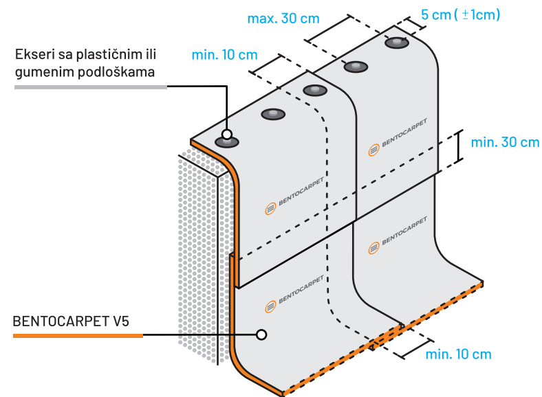
Slika 5. / BENTOCARPET V5, uzdužni preklop na vertikalnom zidu
