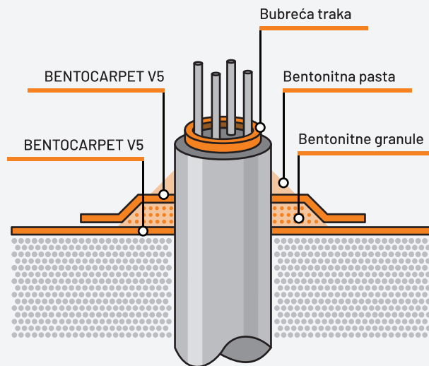
Slika 3. / BENTOCARPET V5, vertikalni proboj
