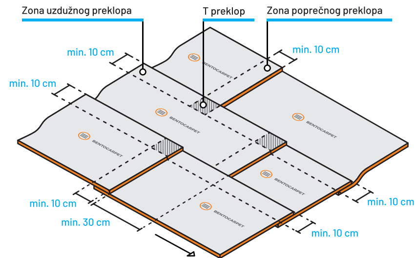
Slika 6. / BENTOCARPET V5, prikaz preklapanja
